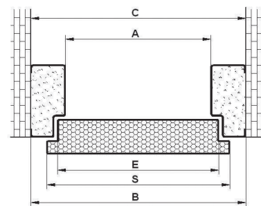
Rysunek poglądowy dla ościeżnic: FC SL, FR SL, FA SL
