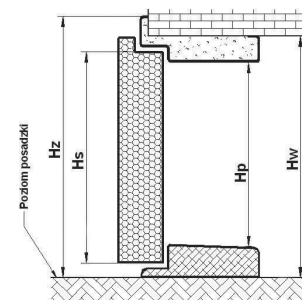
Rysunek poglądowy dla ościeżnicy, drzwi i progów: FT SL
