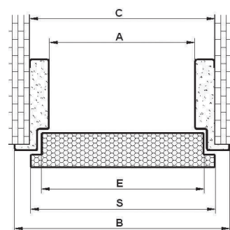
Rysunek poglądowy dla ościeżnic: FT SL
