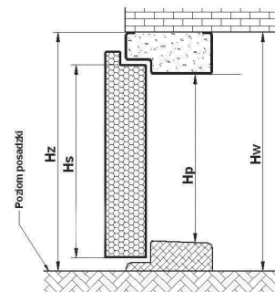
Rysunek poglądowy dla ościeżnic, drzwi i progów: FC SL, FR SL, FA SL
