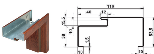
OŚCIEŻNICA ASYMETRYCZNA Z USZCZELKĄ FA SL (do drzwi WX 20, CX 20, SX 20, GSX, GWX 20)
