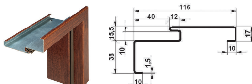
OŚCIEŻNICA NAROŻNIKOWA Z USZCZELKĄ FT SL (do drzwi WX 20, CX 20, SX 20, GSX, GWX 20)
