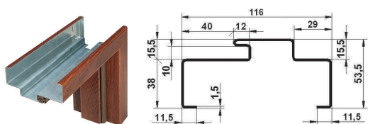
OŚCIEŻNICA SYMETRYCZNA Z USZCZELKĄ FC SL (do drzwi WX 20, CX 20, SX 20, GSX, GWX 20)
