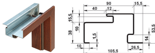
OŚCIEŻNICA ASYMETRYCZNA PORTALOWA Z USZCZELKĄ FR SL (do drzwi WX 20, CX 20, SX 20, GSX, GWX 20)
